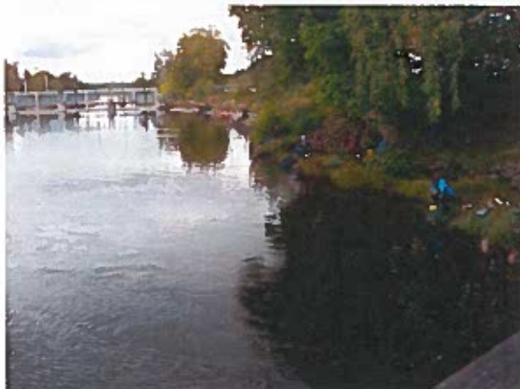
Kolbäcksån, Fagersta
