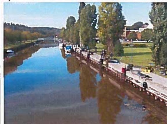
Söderhamnsån
