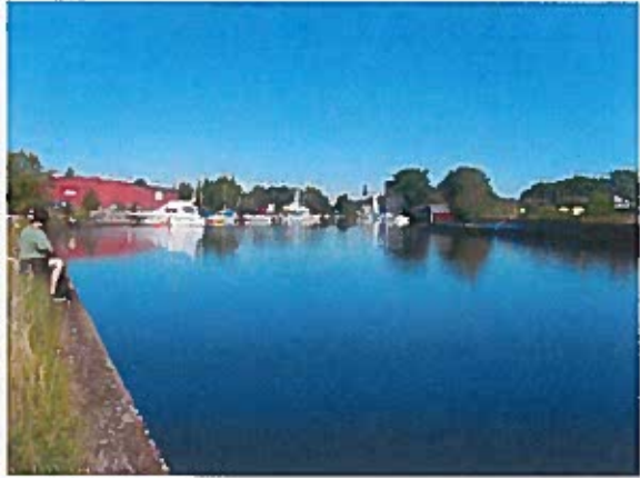
Köpings Hamn
