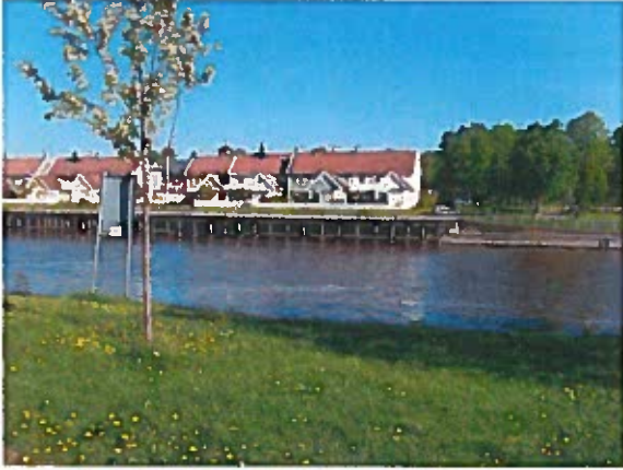
Arbogaån
